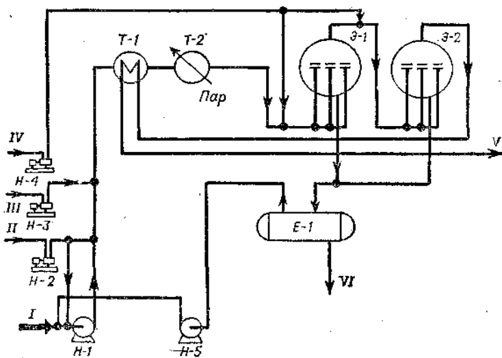
4-сурет. Мұнайды электрлі тұзсыздандыру қондырғысының сұлбасы: I-шікі мұнай; II-деэмульгатор; III-сілті; IV-таза су; V-тұзсызданған мұнай; VI-канализацияға берілетін су;
