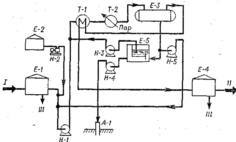
3-сурет. Мұнайды қысыммен термохимиялық сусыздандыру қондырғысының сұлбасы: I-шікі мұнай; II-сусызданған мұнай; III-су;
